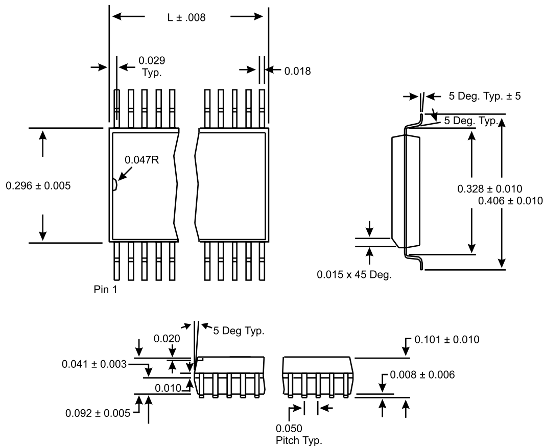
SOIC Package
